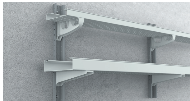
Perfil Omega perfurado disponível em: · Aço galvanizado com revestimento epoxy cinz. · Aço inox AISI 304 com revestimento epoxy cinz. Com suportes horizontais isolantes U48X
