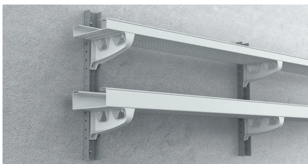
Perfil U perfurado isolante disponível em: · Aço galvanizado com revestimento epoxy cinz. · Aço inox AISI 304 com revestimento epoxy cinz.
