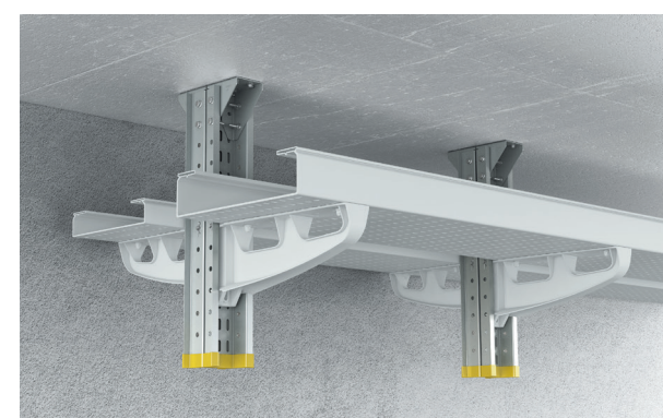
Perfil Omega perfurado disponível em: · Aço inox AISI 304 com revestimento epoxy cinz. · Aço galvanizado com revestimento epoxy cinz. Com suportes horizontais isolantes em U48X
