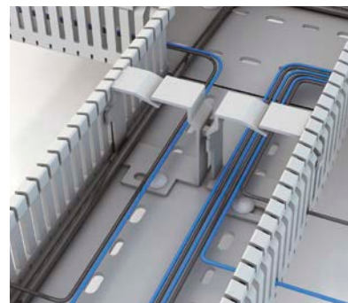
Retentor: permite a ordenação de circuitos. Só 6 referências para 12 dimensões de calha.
