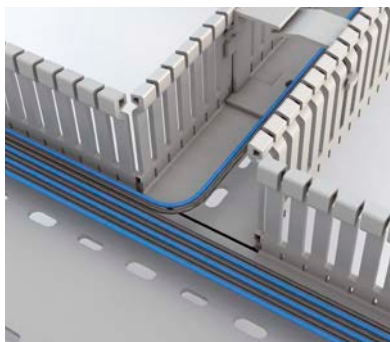
Corte limpo da lateral até à base. Optimização do espaço em derivações. Não danifica o isolamento do cabo.
