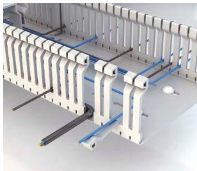
Linguetas flexíveis e resistentes: não se partem acidentalmente.
